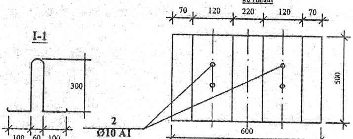
Ø159 mm gaz quvuri uchun temir beton tayanchning yuqoridan ko'rinishi
