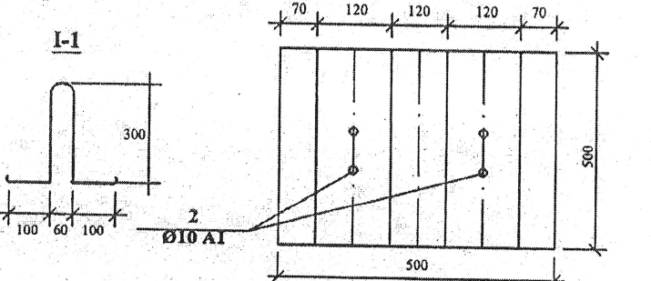
Ø102 mm gaz quvuri uchun temir beton tayanchning yuqoridan ko'rinishi
