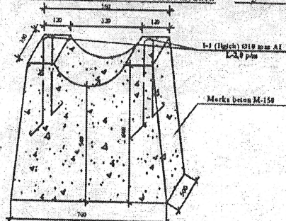
Ø219 mm gaz quvuri uchun temir beton tayanch
