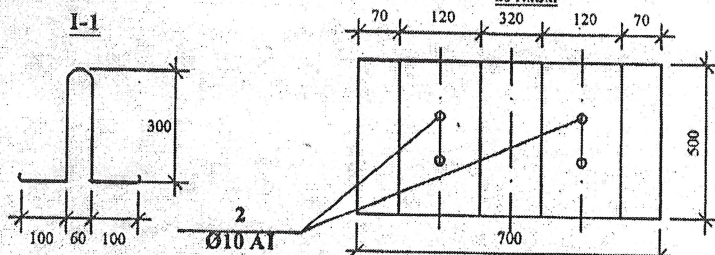
Ø219 mm gaz quvuri uchun temir beton tayanchning yuqoridan ko'rinishi
