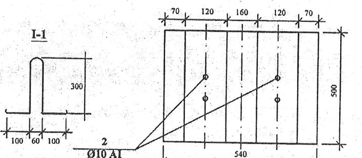
Ø114 mm gaz quvuri uchun temir beton tayanchning yuqoridan ko'rinishi
