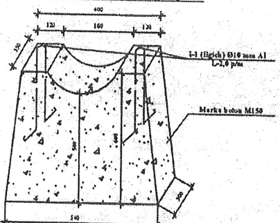
Ø114 mm gaz quvuri uchun temir beton tayanch
