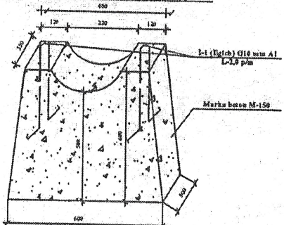
Ø159 mm gaz quvuri uchun temir beton tayanch
